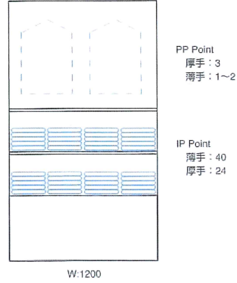
壁面ニッチ フェイスアウトバーがある 棚の場合
