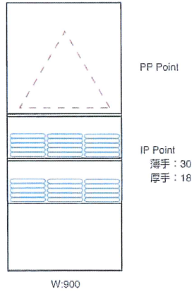
壁面ニッチ (w900) フェイスアウトバーがない 棚の場合
